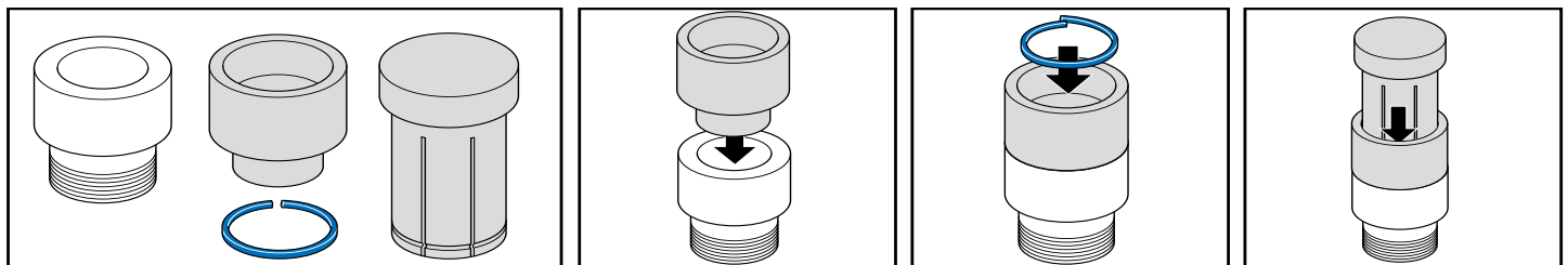
Fitting guide elements | Assemblage éléments de guidage | Elementos de guía de instalación | Instalação de elementos guia
